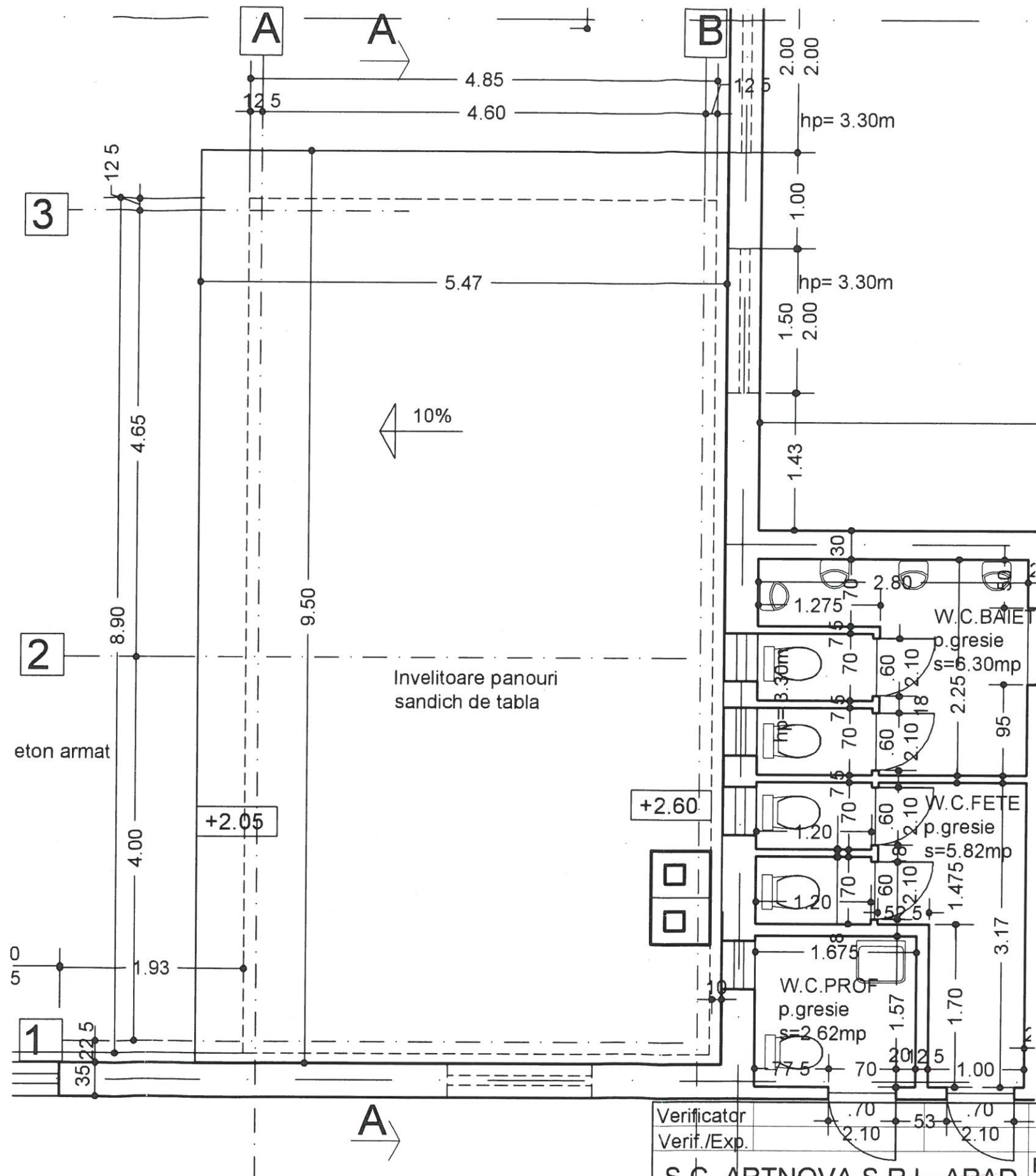
PLAN INVELITOARE COTA + 2.60
