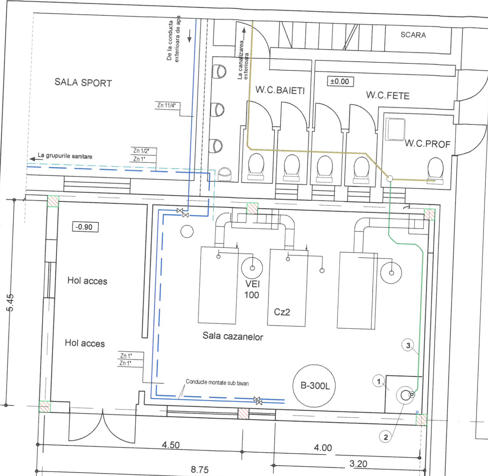
PLAN PARTER CENTRALA TERMICA -SCARA 1:50
